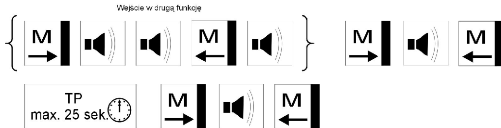
Rys.3 Ustawianie czasu działania przekaźnika TP
