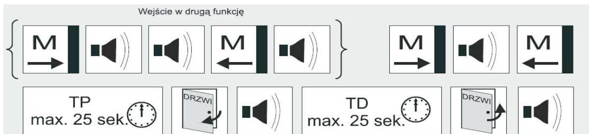
Rys.4 Ustawianie czasu działania TP i TD
